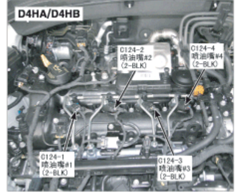
21. 发动机顶部
