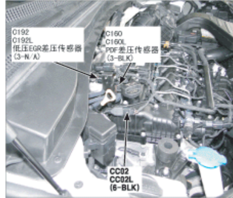
23. 发动机后右
