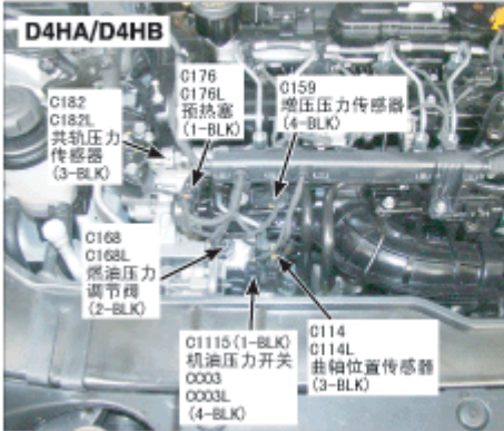
22. 发动机前右
